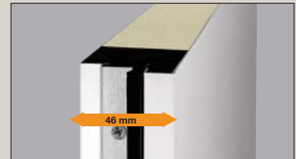
Thermisch getrenntes Türblatt
